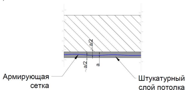
Рис. 13. Армированный штукатурный слой в местах стыка разных материалов и плит перекрытия
